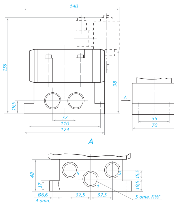
Распределители 211-70; 213-70; 231-70; 233-70
