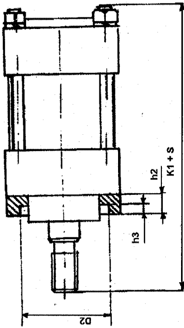
Пневмоцилиндр 1212-D-S
