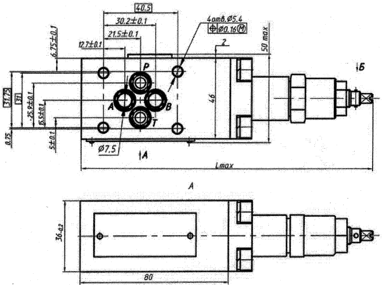
Общий вид с габаритными и присоединительными размерами
